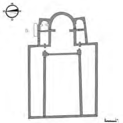
2.- Restitución de la planta del santuario de la basílica
